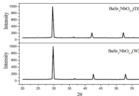
Figure 2: The XRD patterns for BaSr 2 NbO 5.5 (D) and BaSr 2 NbO 5.5 (W).
